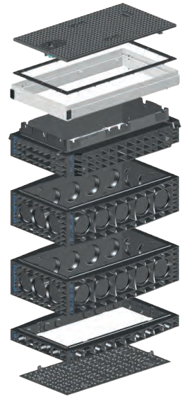
Modularer Aufbau: EK378, Lichtes Maß 400 x 800 mm Abdeckung aus Gusseisen
