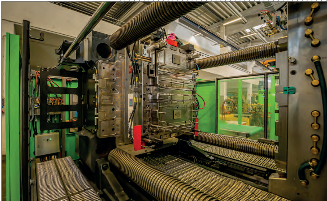
▲ Spritzguss
