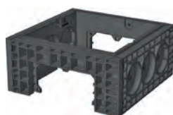
Rahmen 220 mm überbaubar Art.-Nr.: 06 358 0073E 3 x Ø 110 1 x Rechteck Gewicht: 7,0 kg
